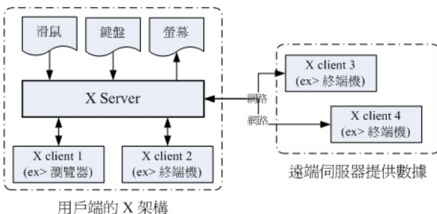
图23.1.1、X Window
