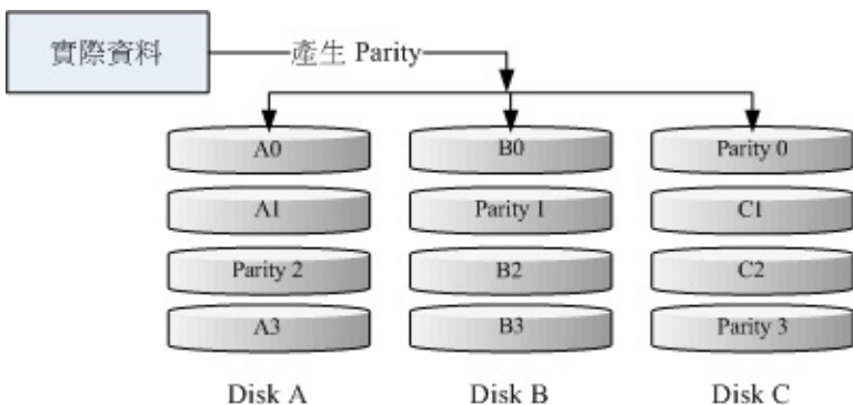
图14.2.4、RAID-5 的磁盘写入示意
