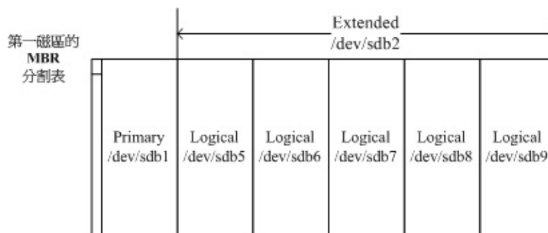
图2.2.6、分区
