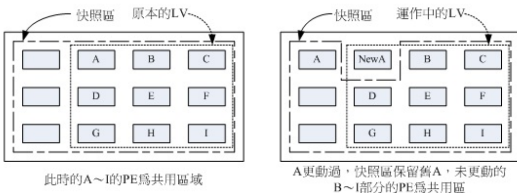
图 14.3.3、LVM
